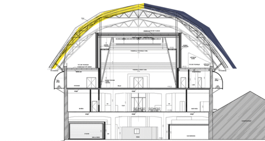
Coupe transversale : salle de musique, Construire-Patrick Bouchain, La Rochelle
