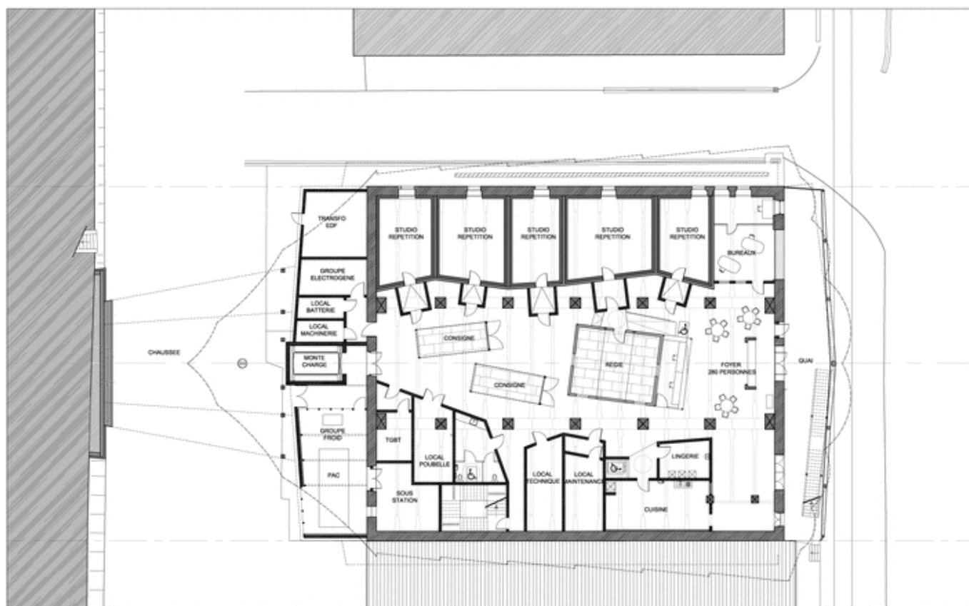
Plan du rez-de-chaussée (niveau port) : salle de musique, Construire-Patrick Bouchain, La Rochelle
